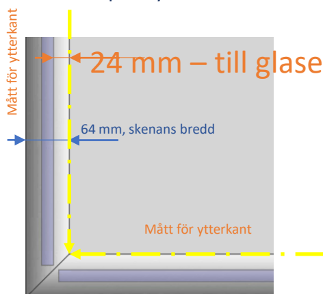
Princip för ytterhörn
