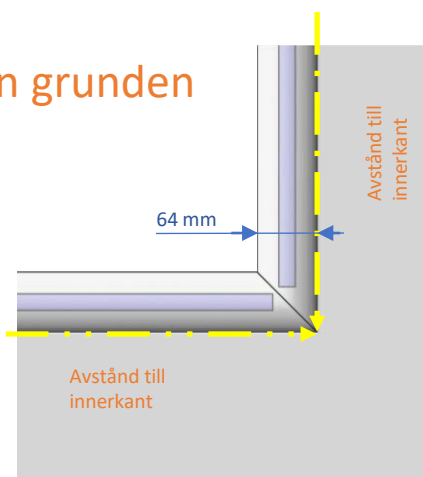
Princip för innerhörn
